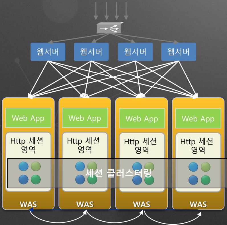
WAS를 이용한 클러스터링
